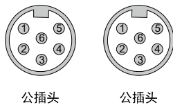
双M16, 6芯针脚俯视图 (传感器端)
